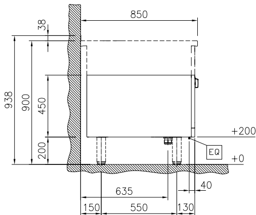
Zij aanzicht
